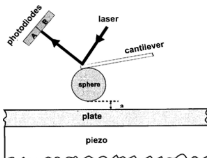
Hình 3: Sơ đồ hệ đo lực Casimir giữa quả cầu và tấm bằng kính hiển vi nguyên tử lực
