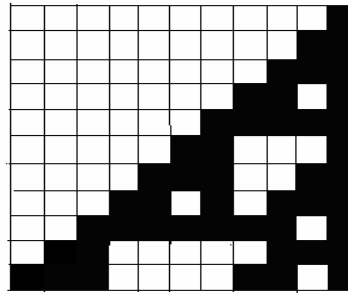
Hình 4.1. Kết quả áp dụng 110 sau 10 lần lặp
