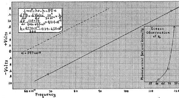
Hình 2. Hiệu ứng quang điện cho phép chúng ta xác định tỉ số h/e , chỉ là độ dốc của đường biểu diễn Volts vs. tần số. Đồ thị trên là dữ liệu của Millikan xác định h/e = 4.134^{15} (đơn vị cgs) với sai số là 1%. Ở đây ta thấy h & e đi đôi với nhau. Ngay cả trong các phép đo hiện đại, ta sẽ thấy việc đo đạc h sẽ còn tiếp tục tùy thuộc vào giá trị của e .
