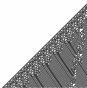
Hình 4.2. Kết quả áp dụng quy tắc 110 sau 700 lần lặp
