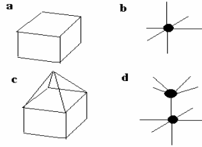
Hình 2.1. Diện tích, thể tích và biểu diễn trên mạng spin
