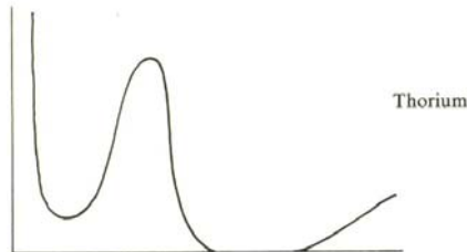
Tiết diện hấp thụ neutron của Th232
